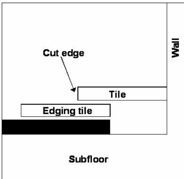
Cut edge of the edge modules
